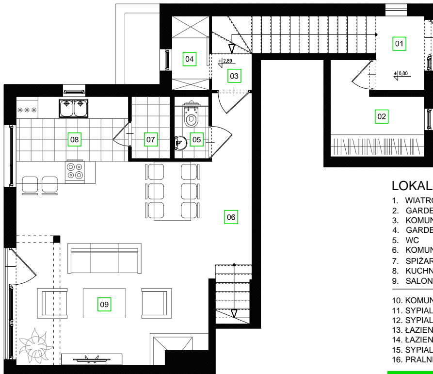
RZUT I PIĘTRA + PARTER
