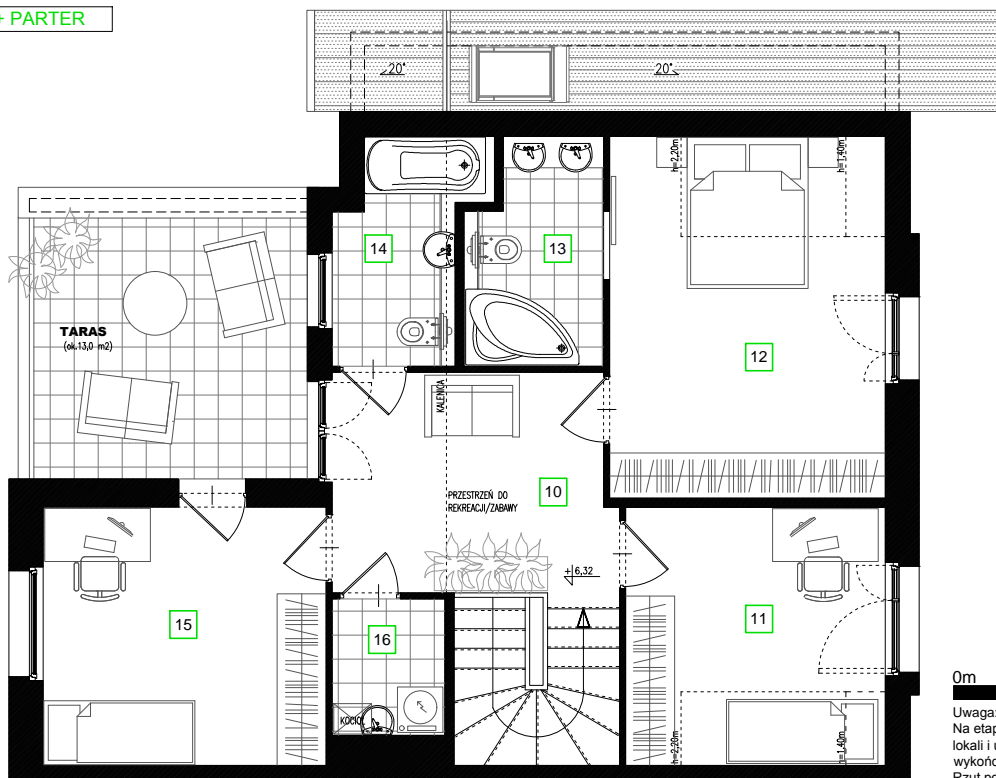
RZUT II PIĘTRA-PODDASZE
